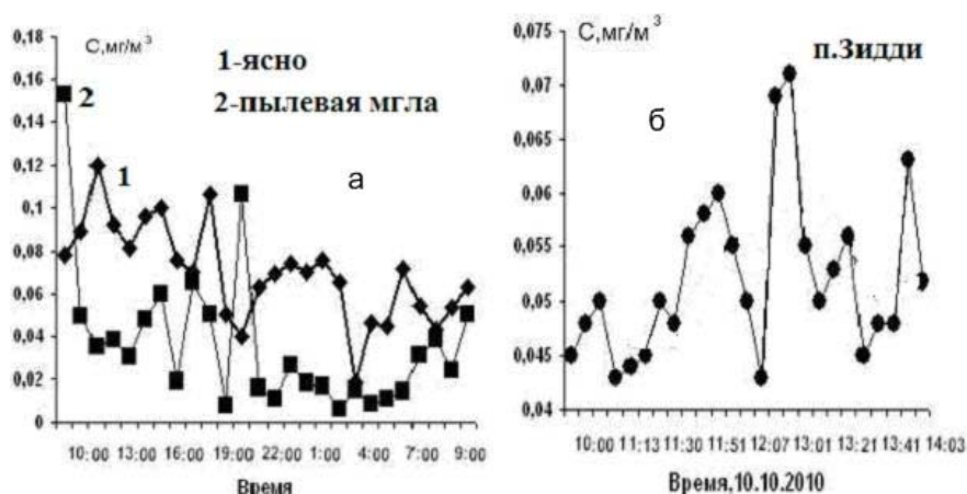
Рис.3. а-Изменение суточной концентрации O_3 в ясной атмосфере и в период пылевой мглы в г.Душанбе. б-Изменение концентрации O_3 в дневное время в п. Зидды (экспериментальная высокогорная база Института физиологии растений и генетики АН Республики Таджикистан).
