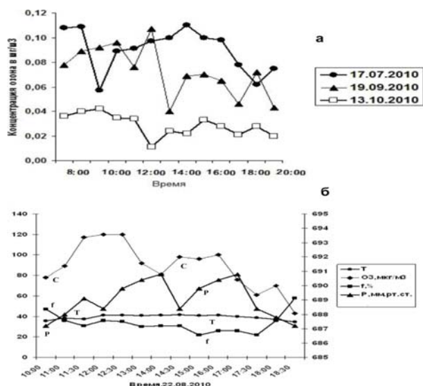
Рис.1. а) Изменение концентрации озона в период июль-октябрь 2010года, б) Изменение концентрации О 3 , температуры, давления и влажности воздуха в течение 22 августа 2010 года в г.Душанбе
