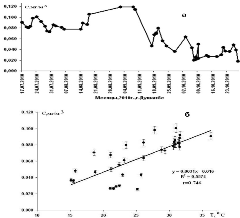
Рис.2. Изменение концентрации O_3 в июле-октябре 2010г. в г.Душанбе.
