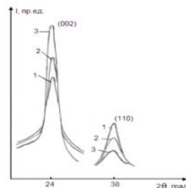
Рис. 5. Дифрактограммы пленок CdTe толщиной 110 мкм подвергнутых отжигу. 1 – исходный; 2 – T_{\text{отж}}=523 ; 3 – 603К
