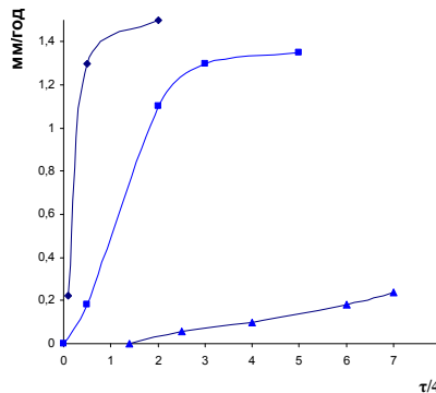
Рис.2. Изменение скорости коррозии в о времени для Ст.3 в 3%-м растворе NaCl (10% ГРМ в ДШФВН) при t= 60 °С и n , мин -1 ; 1-500; 2-1000; 3-2000
