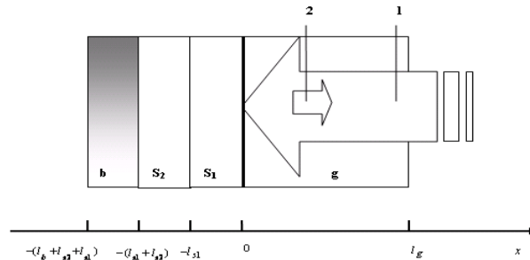
Рис.1. Геометрия задачи для двухслойных образцов в ФА - ячейке для случая, когда первый слой является сильнопоглощающим: 1- падающий на поверхность первого слоя луч, 2- отраженная от неё часть луча, g, S 1 , S 2 , b –соответственно газ, первый слой, второй
