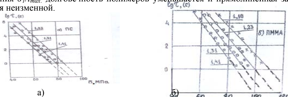
Рис.2. Зависимость логарифма долговечности ( \lg \tau ) для ПС (а) и для ПММА (б) от главного нормального напряжения \sigma_1 при различных отношениях \sigma_1/t_{\max} : а- ПС:1-1,23; 2-1,31; 3-1,41; б - ПММА:1-1,10; 2-1,23; 3-1,31; 4-1,41.
