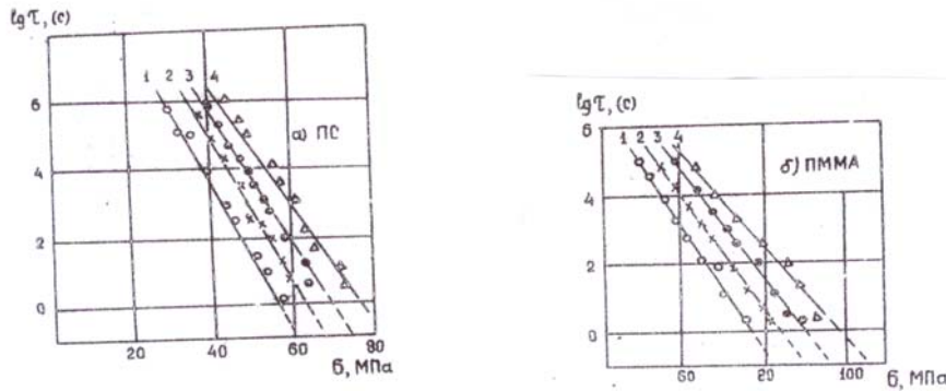
Рис.1. Зависимость логарифма долговечности ( \lg \tau ) для ПС (а) и для ПММА (б) от напряжения \sigma при растяжении (1), кручении (2), изгибе (3) и совместном действии растяжения с кручением (4), когда \sigma_1/t_{\max} = 1,21 .
