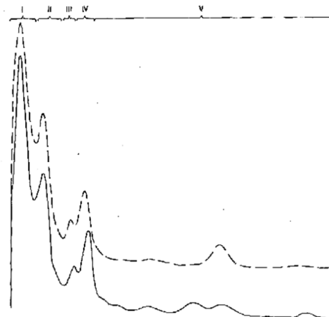
Рис. 1. Денситограмма при 672 нм после электрофореза обработанных дигитонином хлоропластов хлопчатника сорта 108-Ф (сплошная линия) и мутанта Дуплекс (штриховая линия). Цифрами обозначены номера электрофоретических зон.
