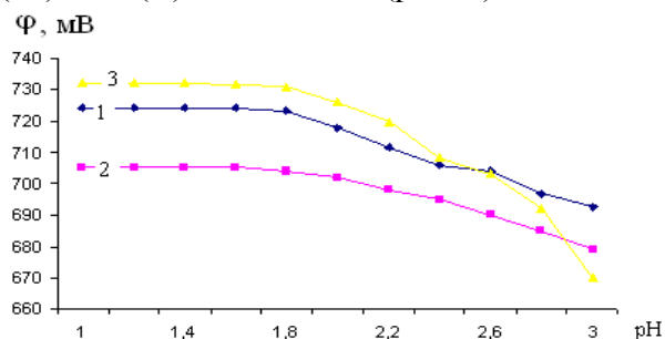
Рис.1. Зависимость окислительного потенциала φ от рН раствора. Т=298К, J=0,5 моль/л. Кривые относятся к следующим фоновым электролитам:
