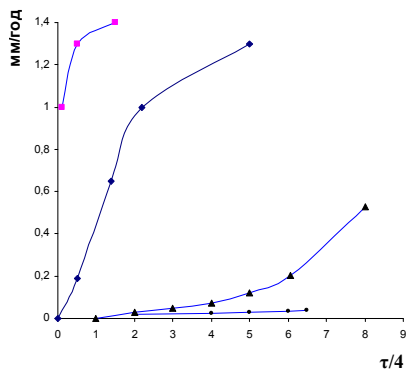
Рис.1. Изменение скорости коррозии ( \rho ) в зависимости от времени ( \tau ) в 3%-м растворе NaCl при n=1000 мин -1 и t , °С: 1-40; 2-50; 3-60; 4-70; (10%-й раствор ГРМ в ДШФВН)
