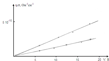
Рис. 6. Начальный участок вольтамперной характеристики пленок CdTe.
