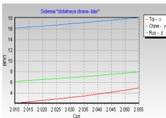
Рис. 4. Результаты компьютерных экспериментов при a=0,1 .
