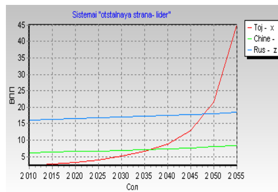
Рис. 5. Результаты компьютерных экспериментов при a=0,5 .
