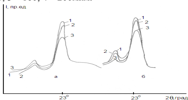
Рис. 2. Дифрактограммы пленок CdTe при различных толщинах а) CdTe-CdTe; б) CdTe-GaAs: 1-80, 2-110, 3-200 мкм
