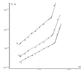
Рис. 4. Влияние температуры отжига на проводимость пленок при D=110\text{мкм} ; 1 – исходный, 2 – T_{\text{отж}}=523\text{К} , 3 – 603К
