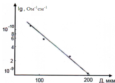
Рис. 3. Зависимость проводимости от толщины пленок.
