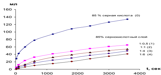
Рис. 5. Зависимость объема выделившегося CO 2 от весового соотношения компонентов (0 -85%-серная кислота; 1- 85% сернокислотный слой, полученной при соотношении серной кислоты и ДШФВН 1- 1:0,5; 2 - 1:1; 3 - 1:4; 4 - 1:6) и от времени взаимодействия смеси серной кислоты и ДШФВН с карбонатными породами
