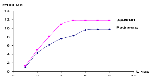
Рис. 3. Зависимость растворения парафин-асфальтено-смолистых отложений в ДШФВН и ее рафинаде от времени в стационарных условиях.
