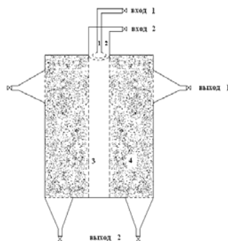
Рис.1. Модель скважины для изучения образования сернокислотного экстракта и рафинада при одновременно – раздельной закачке серной кислоты и ДШФВН. 1-НКТ; 2-обсадная колонна; 3-перфорация; 4 – пласт.
