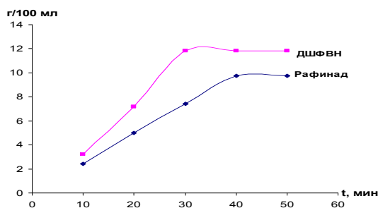
Рис. 4. Зависимость растворения парафин-асфальтено-смолистых отложений в ДШФВН и ее рафинаде от времени в динамических условиях.
