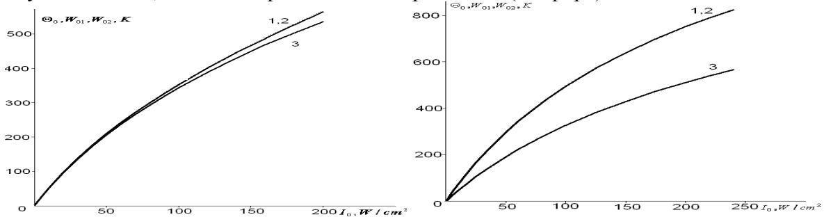
Рис.3. а). Зависимость приращения температур \Theta_0 (кривая 1), W_{01} (кривая 2) и W_{02} (кривая 3) от интенсивности падающего луча для двухслойной системы воздух – кварцевое стекло – сапфир – плавленый кварц. б). Эти же зависимости для двухслойной системы воздух –сапфир-кварцевое стекло- оксид циркония
