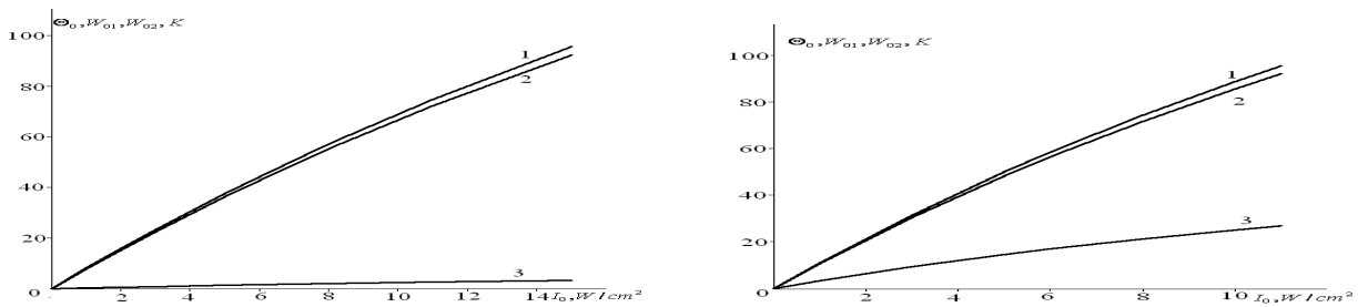
Рис.2. а). Зависимость приращения температур \Theta_0 (кривая 1), W_{01} (кривая 2) и W_{02} (кривая 3) от интенсивности падающего луча для двухслойной системы воздух – ПММА- ПЭНП- нержавеющая сталь. б). Эти же зависимости для двухслойной системы воздух – ПММА- ПЭНП- кварцевое стекло.
