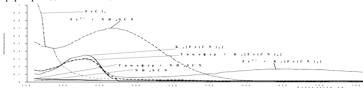
Рис.1. Спектры реагентов, используемых при изучении влияния температуры на физико-химические параметры тимофера и смеси свежеприготовленного тимофера с аналитическими реагентами
