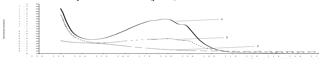
Рис.2. УФ-спектры дипептида изолейцил-триптофан и тимофера после хранения при температурах 35°C и 80°C: 1 - дипептид изолейцил-триптофан, 2 - тимофер после хранения при 35°C, 3 - тимофер после хранения при 80°C.
