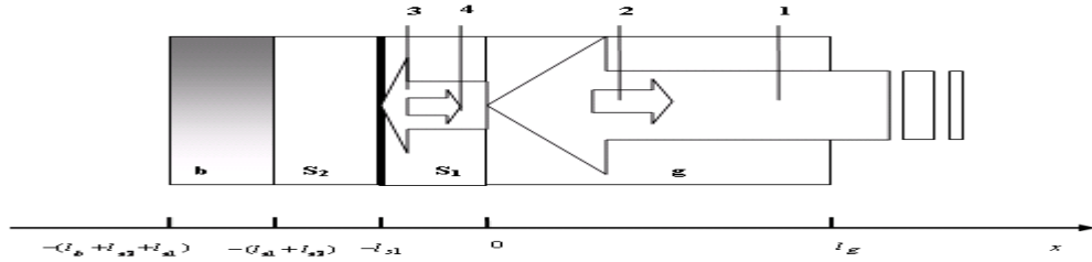
Рис.1. Геометрия задачи для двухслойных образцов в ФА ячейки для случая, когда первый слой является прозрачным, а второй сильнопоглощающим: 1- падающий луч на поверхности первого слоя, 2- отраженная часть луча от поверхности первого слоя, 3- падающая часть луча на поверхности второго слоя, 4- отраженная часть луча от поверхности второго слоя, г, S 1 , S 2 , б – соответственно газ, первый слой, второй слой и подложка.
