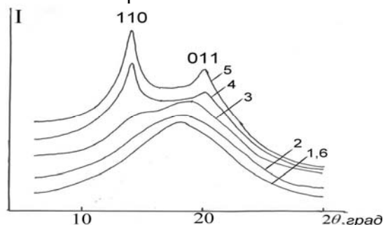
Рис.1. Большеугловые рентгенограммы СКИ-3 при деформировании.
