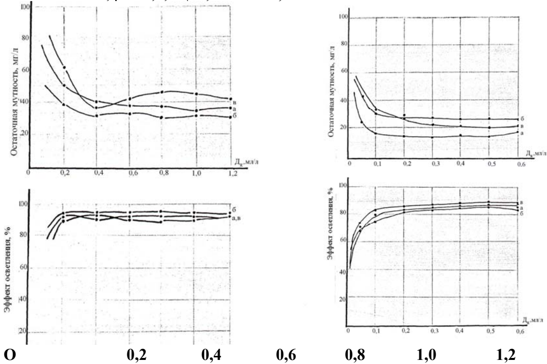
Рис.2. Зависимость остаточной мутности и эффекта осветления от дозы коагулянта
