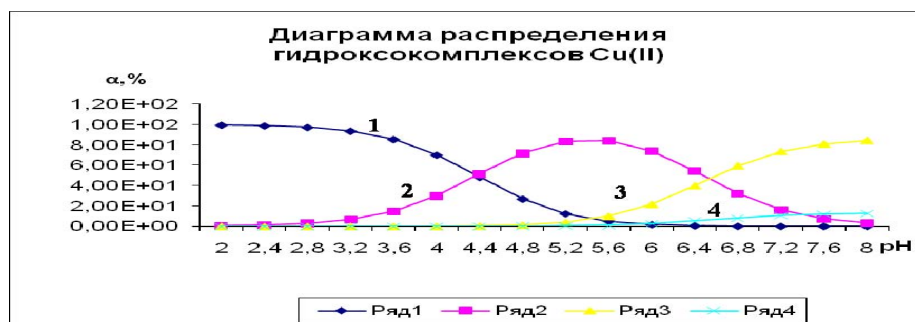
Рис.4. Массовая доля свободных ионов Cu(II) и его гидролизных форм при 318,16 К и J=1,0 моль/л. Кривые относятся к: 1. – [Cu(H 2 O) 4 ] 2+ ; 2. – [CuOH(H 2 O) 3 ] 2+ ; 3. – [Cu 2 (OH) 2 (H 2 O) 4 ] 2+ ; 4. – [Cu(OH) 2 (H 2 O) 2 ] 0 .
