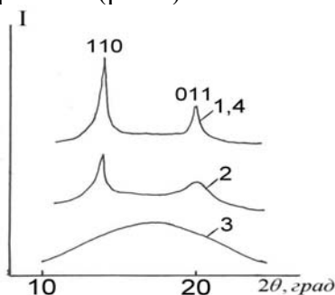
Рис. 4. Большеугловые рентгенограммы деформированного СКИ-3 на \epsilon = 700\% при циклическом температурном воздействии 1 – T = 10; 2 – 50; 3 – 90; 4 – охл. 10^0\text{C} .
