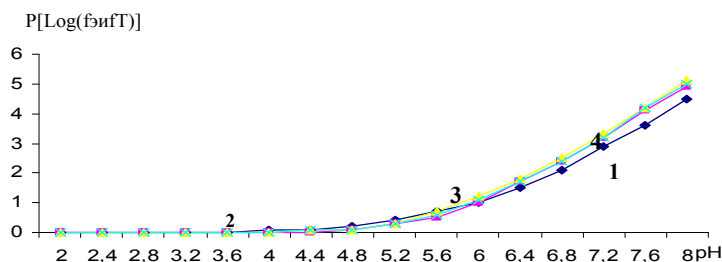
Рис. 3. Зависимость экспериментальной ( f_0 ) и теоретической ( f_T ) окислительной функции от рН в системе: Cu(0)/Cu(II)- H 2 O при T=318,16 К, J=1,0 и C Cu(0) =C Cu(II) =1·10 -4 моль/л. Кривые относятся к: 1 – экспериментальная окислительная функция; 2, 3, 4 – теоретические окислительные функции.
