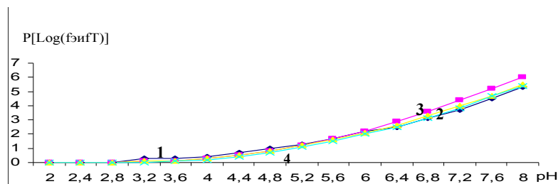
Рис.2. Зависимость экспериментальной ( f_0 ) и теоретической ( f_T ) окислительной функции от рН в системе: Cu(0)/Cu(II)- H 2 O при T=318,16 К, J=1,0 и C Cu(0) =C Cu(II) =1·10 -3 моль/л. Кривые относятся к: 1. – экспериментальная окислительная функция; 2, 3, 4. – теоретические окислительные функции.
