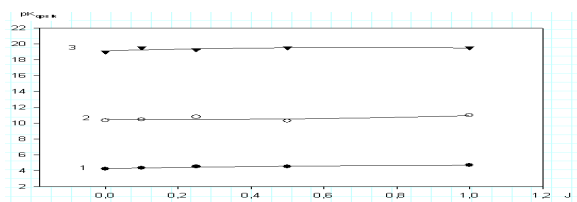
Рис.5. Зависимость констант образования комплексных соединений ( \lg\beta ) от ионной силы J ( 0,1 \div 1,0 ) моль/л, Кривые относятся к: 1 – [\text{CuOH}(\text{H}_2\text{O})_3]^+ ; 2. – [\text{Cu}_2(\text{OH})_2(\text{H}_2\text{O})_6]^{2+} ; 3. – [\text{Cu}(\text{OH})_2(\text{H}_2\text{O})_2]^0 .
