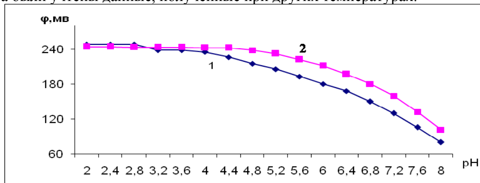
Рис.1 Зависимость окислительного потенциала \phi от рН при 318,16 К, J=1,0 моль/л и концентрациях: [Cu(II)]=1*10 -3 (кривая 1) и 1*10 -4 (кривая 2).
