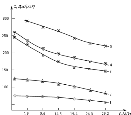
Рис.1. Зависимость удельной изобарной теплоемкости исследуемых образцов от давления при различных температурах: 1- 293 К; 2-303К; 3-313К; 4-323К; 5-353 К.
