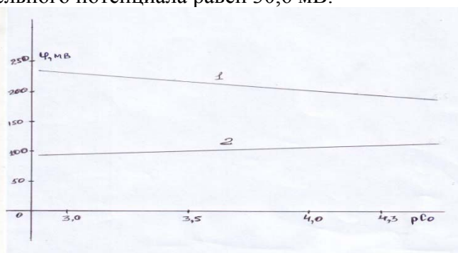
Рис.2. Зависимость окислительного потенциала \phi от p\text{Co} . Кривые относятся к pH: 1 - 5,0; 2 - 8,0.
