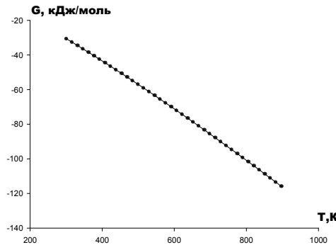
Рис.4. Температурная зависимость энергии Гиббса для магнезия: точки –расчет по формуле (4), сплошная линия- расчет по формуле
