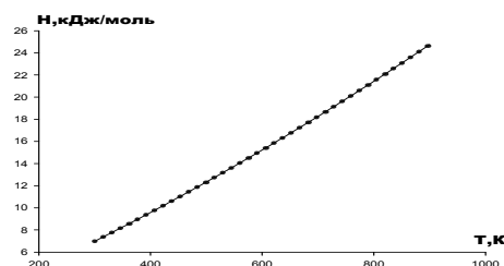
Рис. 2. Температурная зависимость энтальпии для магния: точки – расчет по формуле (2), сплошная линия- расчет по формуле H=0.0415+0.0209T+7.455 \cdot 10^{-6} T^2-1.98 \cdot 10^{-10} T^3 (кДж/моль)
