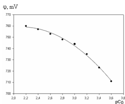
Рис.2. Зависимость окислительного потенциала \varphi от pC_0 . Кривая рассчитана по программе SigmaPlot 10.0, а точки экспериментально измеренные.
