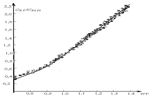
Рис.2. Зависимость относительной теплоемкости \frac{C_{p,T}}{C_{p,T_1}} от относительной температуры \frac{T}{T_1} исследуемых
