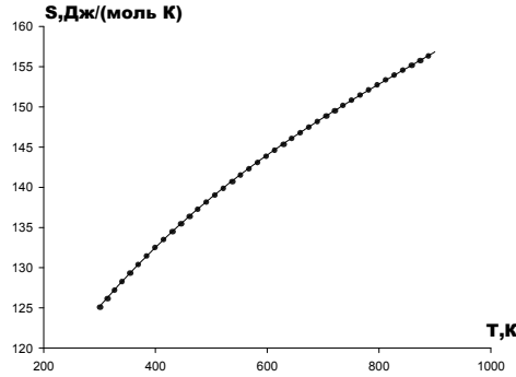
Рис.3. Температурная зависимость энтропии для магнезия: точки- расчет по формуле (3), сплошная линия- расчет по формуле
