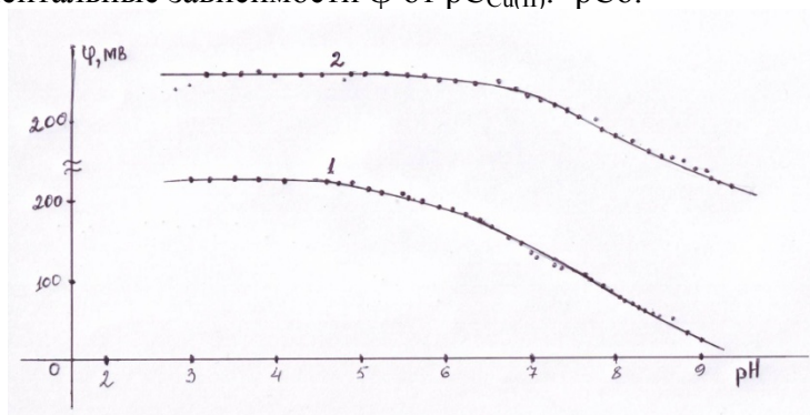
Рис.1 Зависимость окислительного потенциала \phi от pH при 308,16 К, J=0,50 моль/л и концентрациях: [\text{Cu(II)}]=1 \cdot 10^{-3} (кривая 1) и 1 \cdot 10^{-4} (кривая 2)
