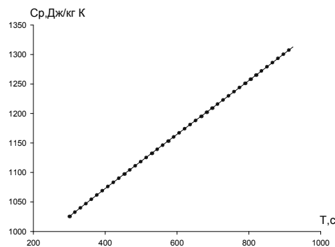
Рис.1. Зависимость C_p(T) магния от температуры T (точка-эксперимент, сплошная линия вычисленная по формуле (1))
